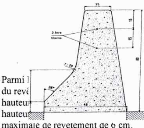
re 3 : type de glissière rigide, la plus importante des deux surfaces inclinées du muret doit être telle que le véhicule soit renvoyé au maximum à 1 m de la face avant.
